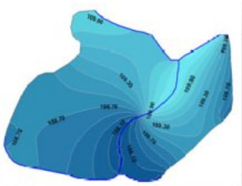
Hladina podzemnej vody - uzatvorené stavidlo na kanáli
