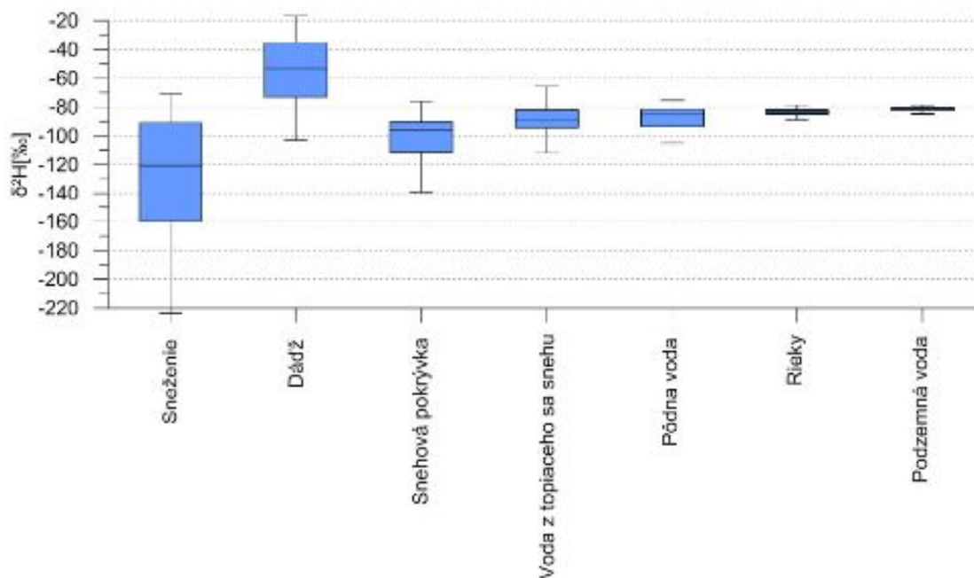
Obr. Rozsah hodnôt \delta^2\text{H} v rôznych častiach hydrologického cyklu spojených so snehom.
